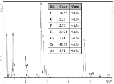
焊盘端断面的元素分析
