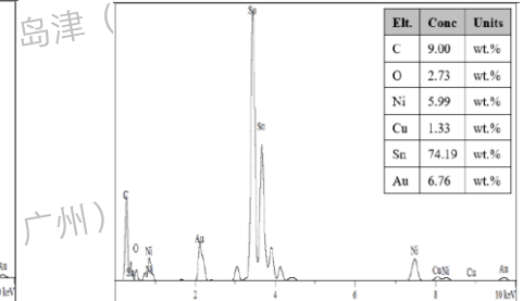
铜柱端断面的元素分析结果
