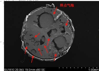
铜柱端的断面
